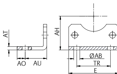
Fußbefestigung KF 13040-80
